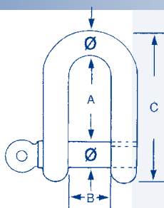
Grillo a cetra in acciaio zincato a caldo
