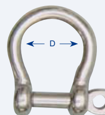
Grillo a cetra in acciaio inox AISI 316
